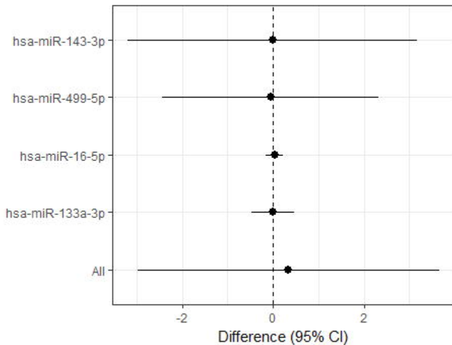
Categorical NRI
