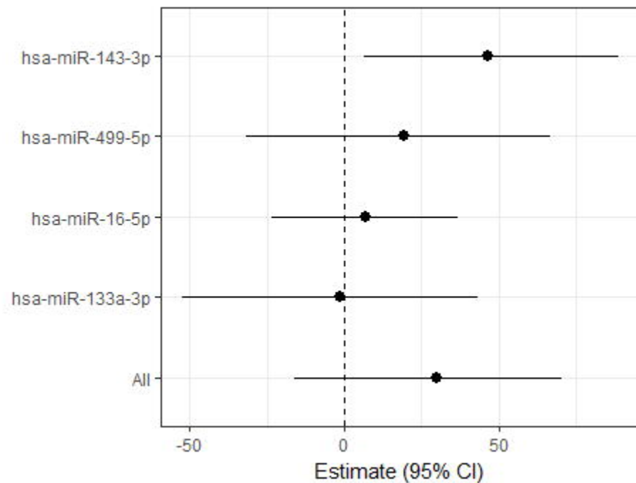
IDI
