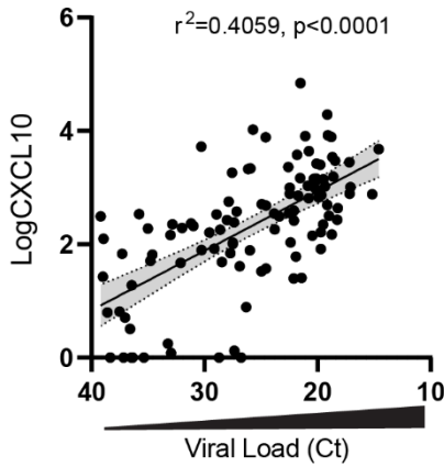
F SARS-CoV-2+
