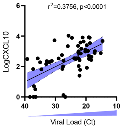
F SARS-CoV-2+
