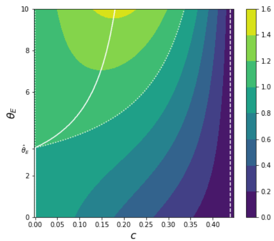
(d) Relative escape pressure \hat{P}_{a'}(c) .
