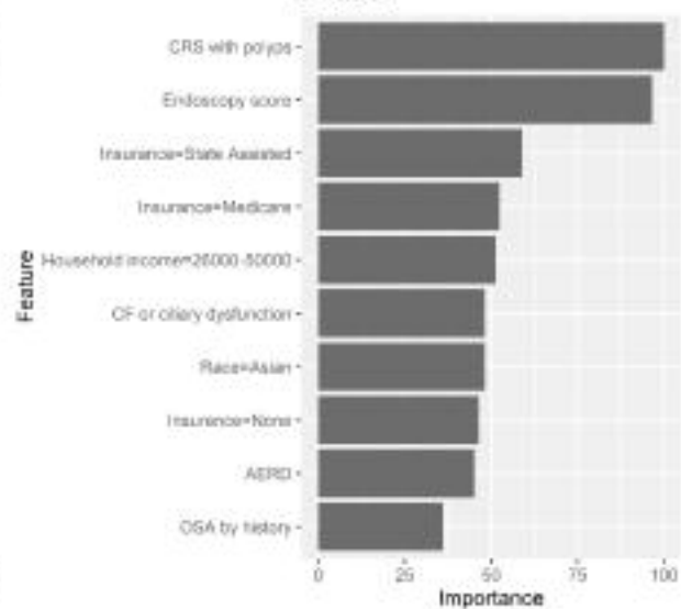
LASSO
