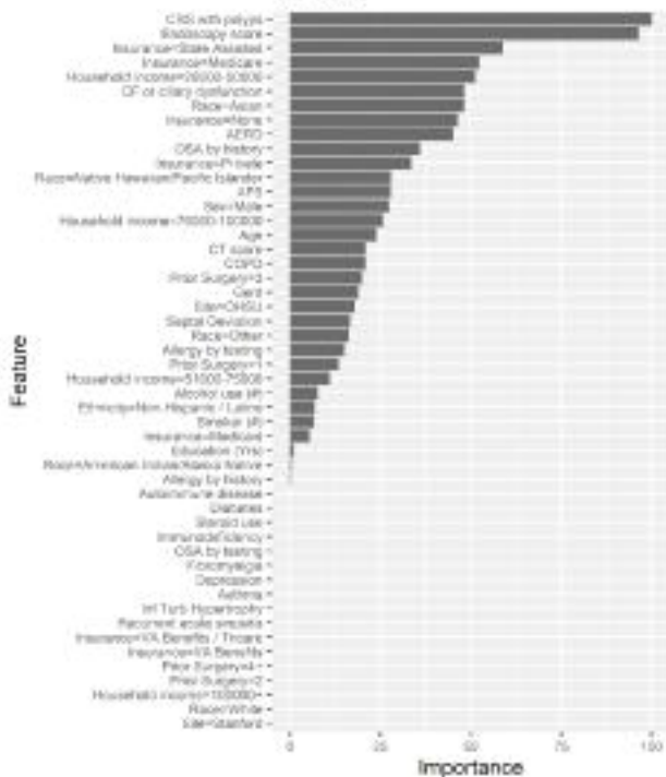
LASSO
