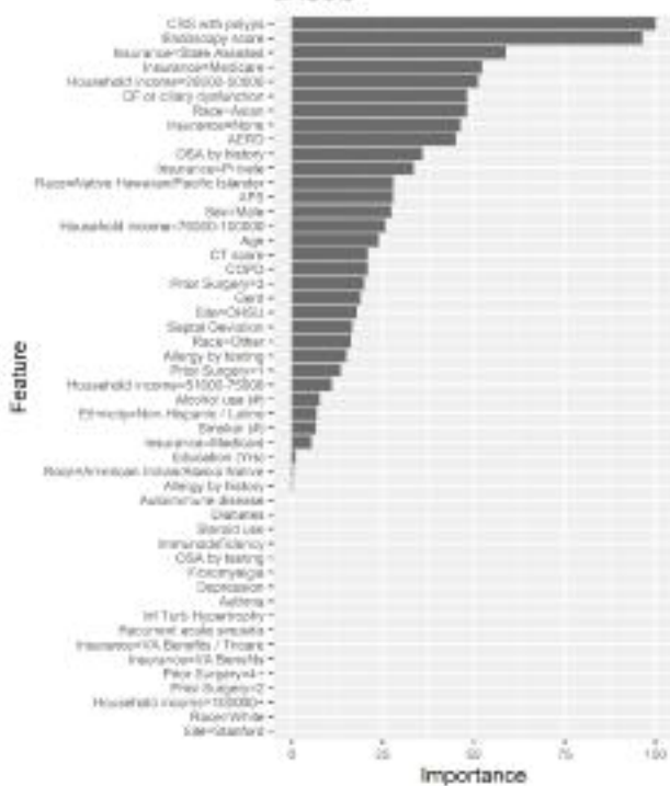
LASSO
