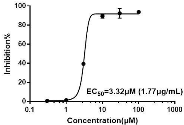
Arbidol
